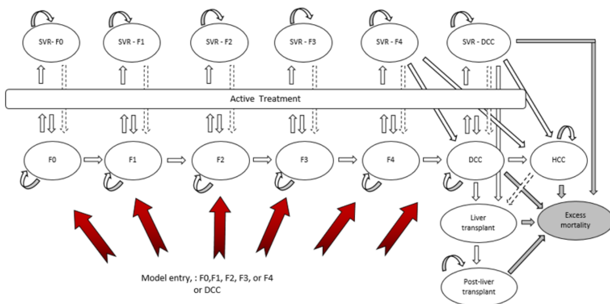
Figur 1 Modellstruktur
